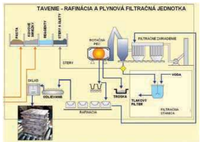
Obr. 5: Tavenie a rafinácia olova
