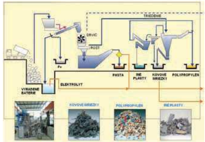
Obr. 4: Drvenie a separácia zložiek olovených akumulátorov
